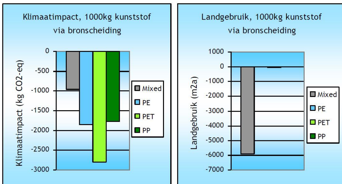
Figuur 19: Klimaatimpact en landgebruik van recycling t.o.v. verbranden van kunststof afval via bronscheiding (CE Delft, 2011)
